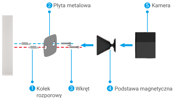
Rys. 2 Mocowanie przy użyciu wkrętów
