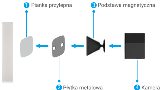
Rys. 1 Mocowanie przy użyciu pianki przylepnej
